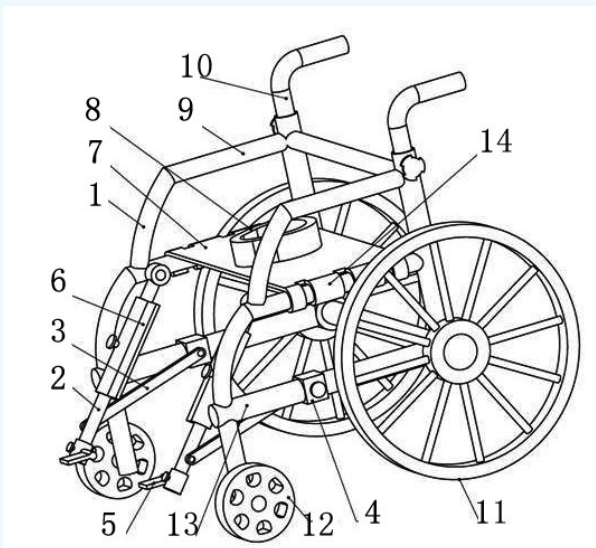
产品示意图
